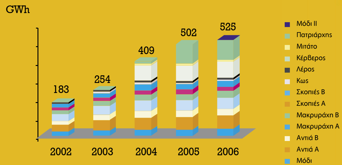
Ηλεκτροπαραγωγή ανά αιολικό πάρκο 2002-2006
