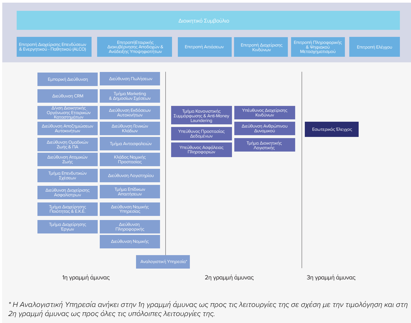
Σχήμα: Πρότυπο τριών γραμμών άμυνας για τη Διακυβέρνηση της Διαχείρισης Κινδύνων
